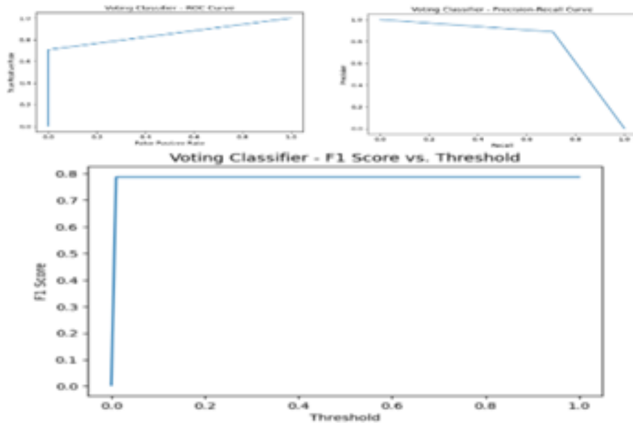
FIGURE 16. F1 score comparison
